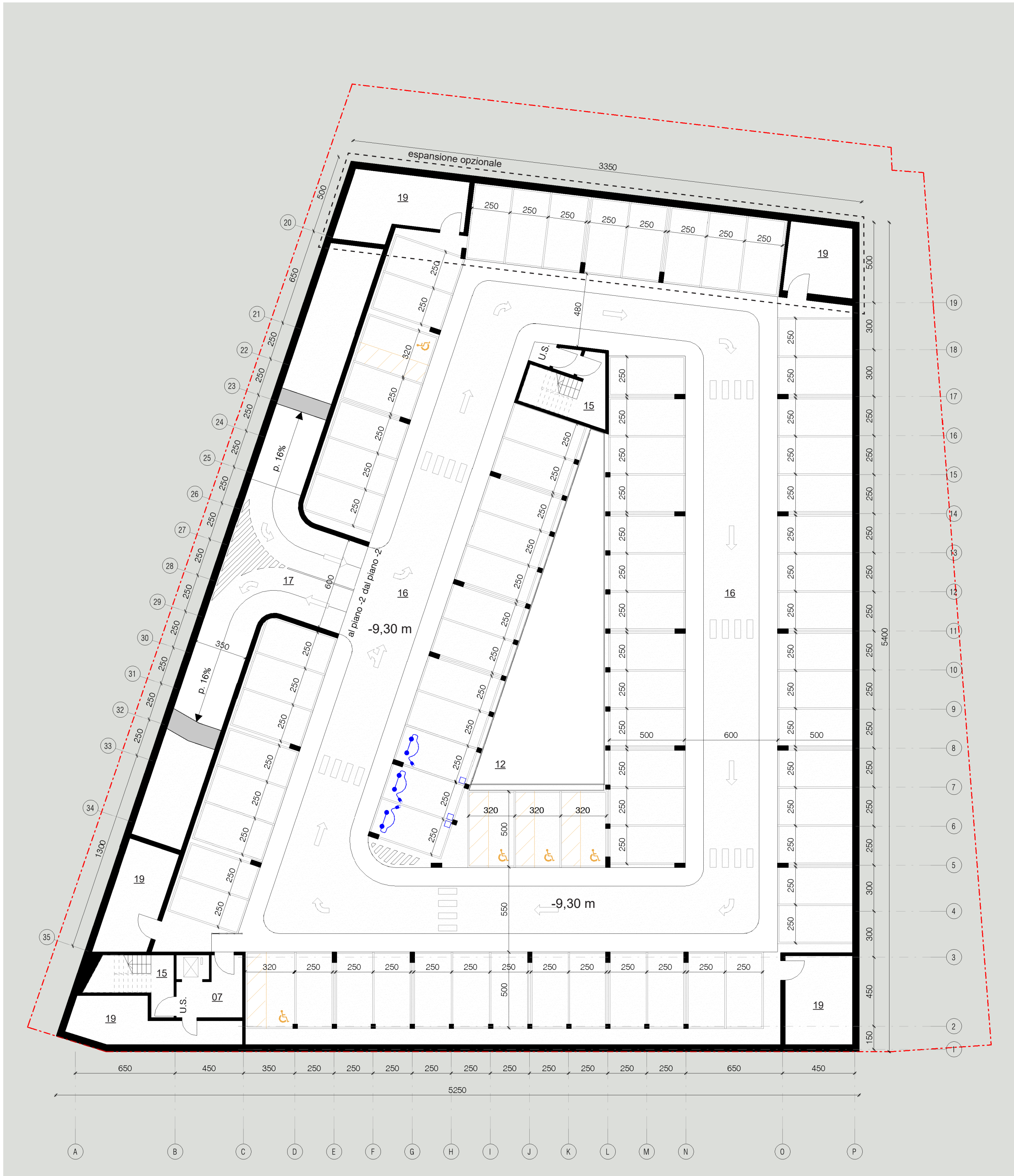
Pianta Livello -3 | 1:200
