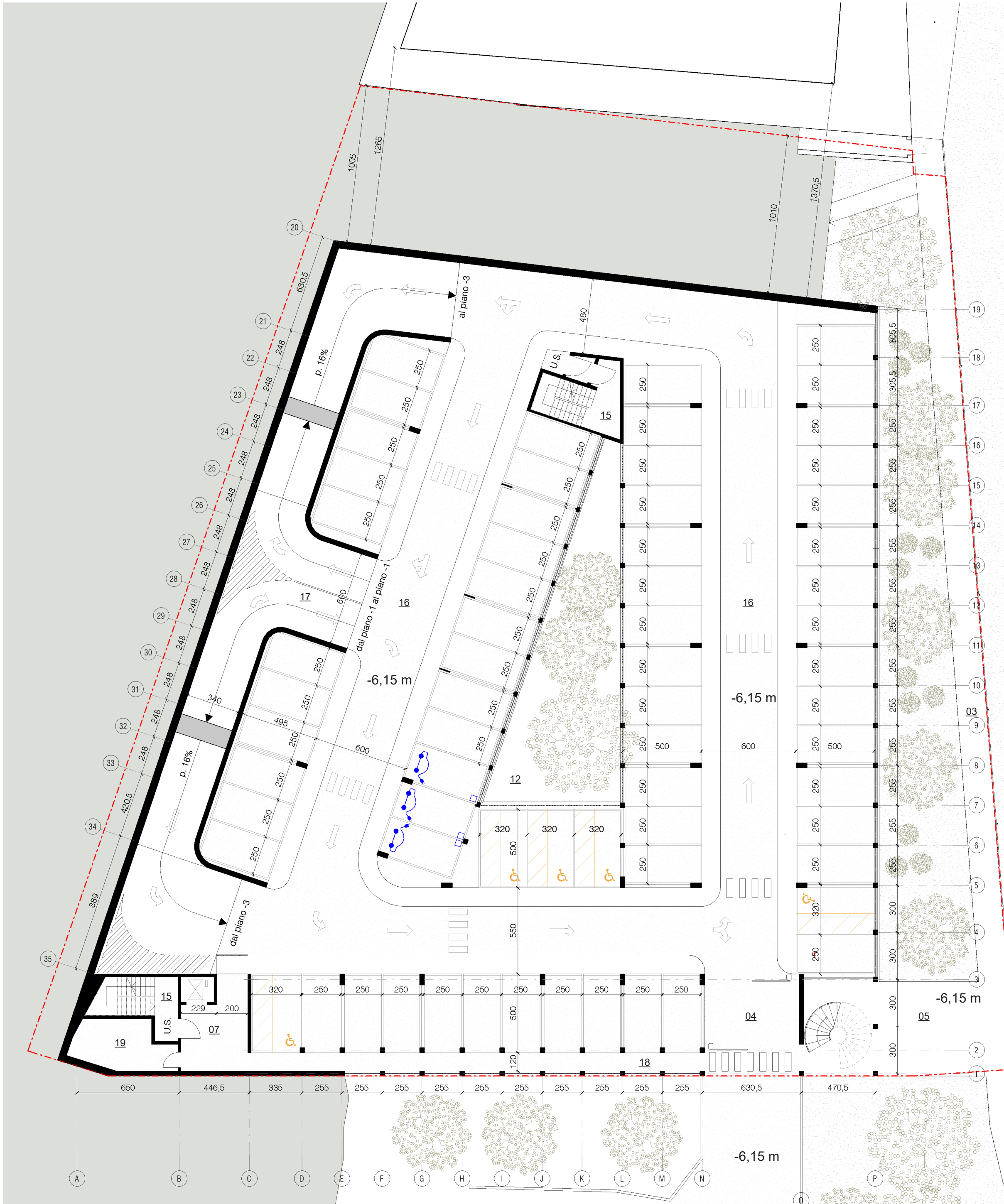
Pianta Livello -2 | 1:200
