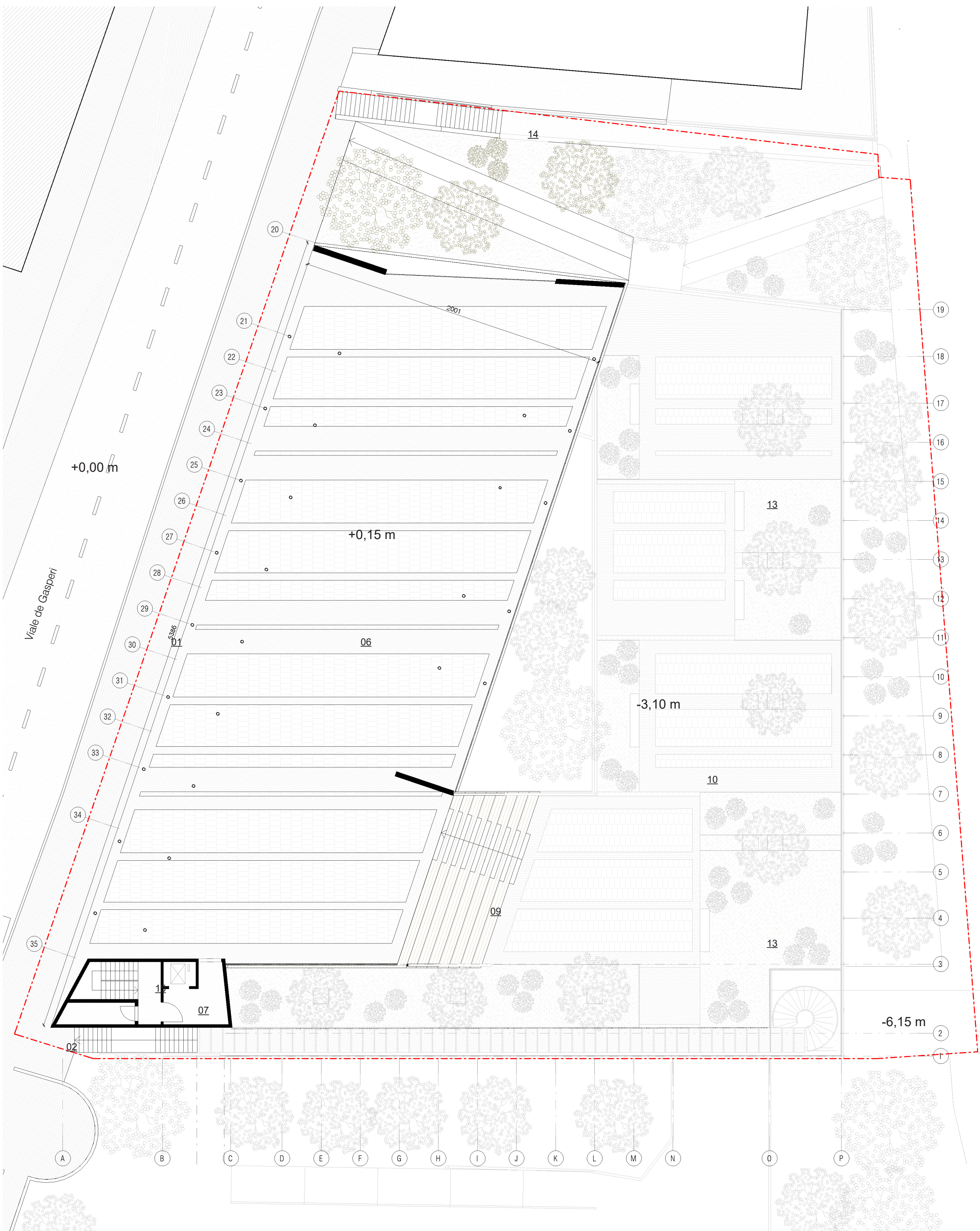
Pianta Livello Strada | 1:200
