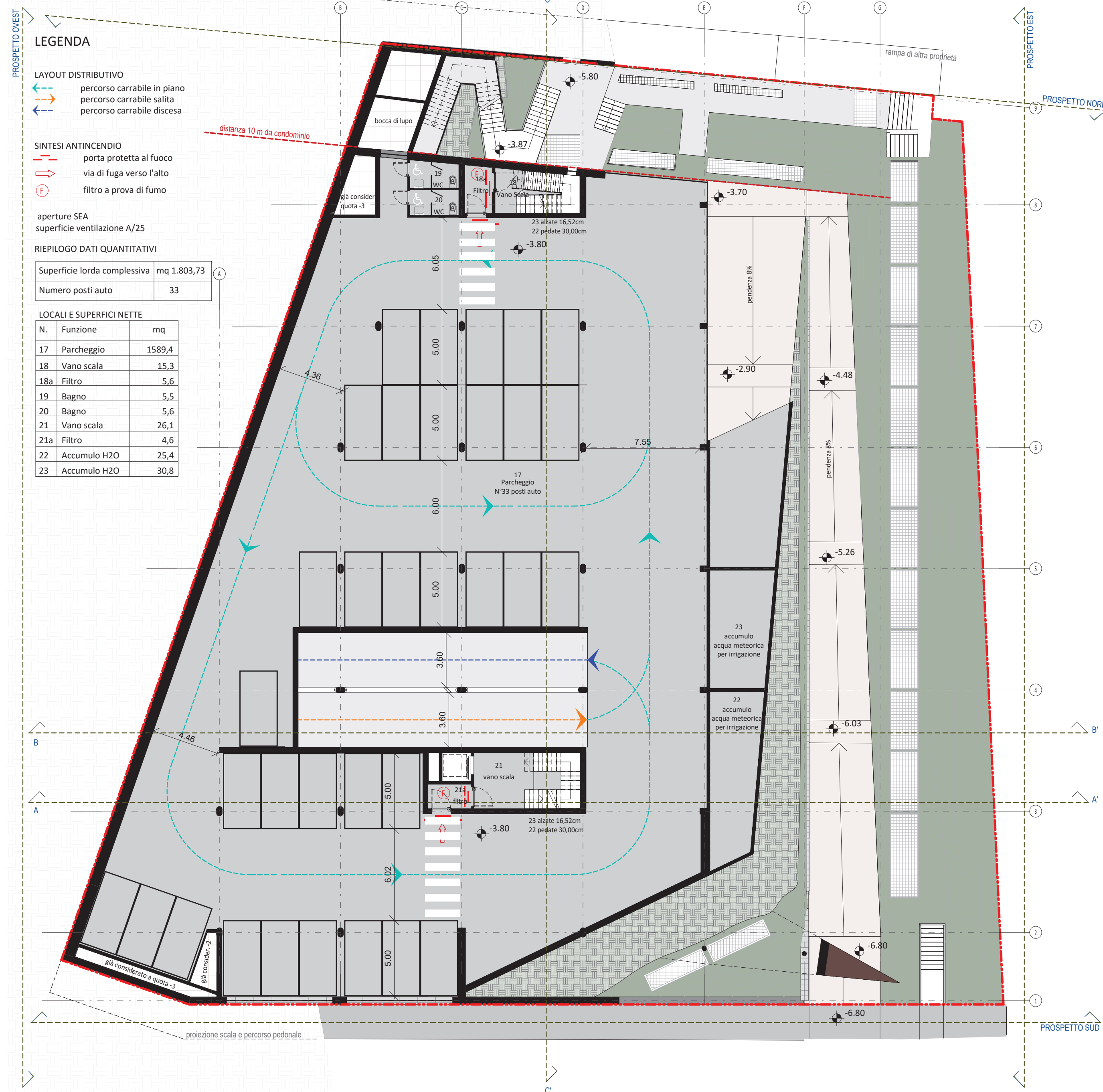
Pianta livello -1 scala 1:200
