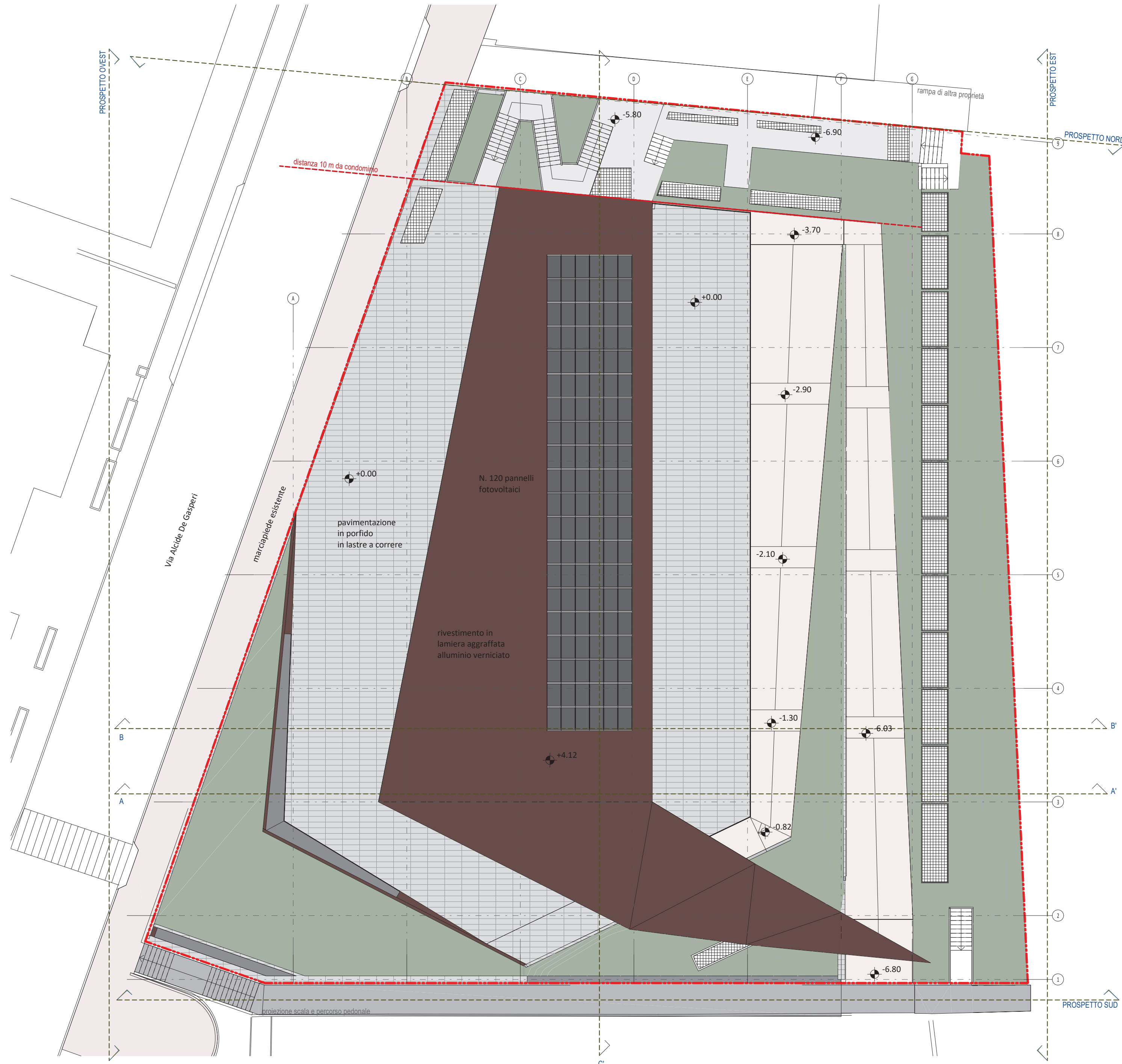
Pianta livello copertura scala 1:200
