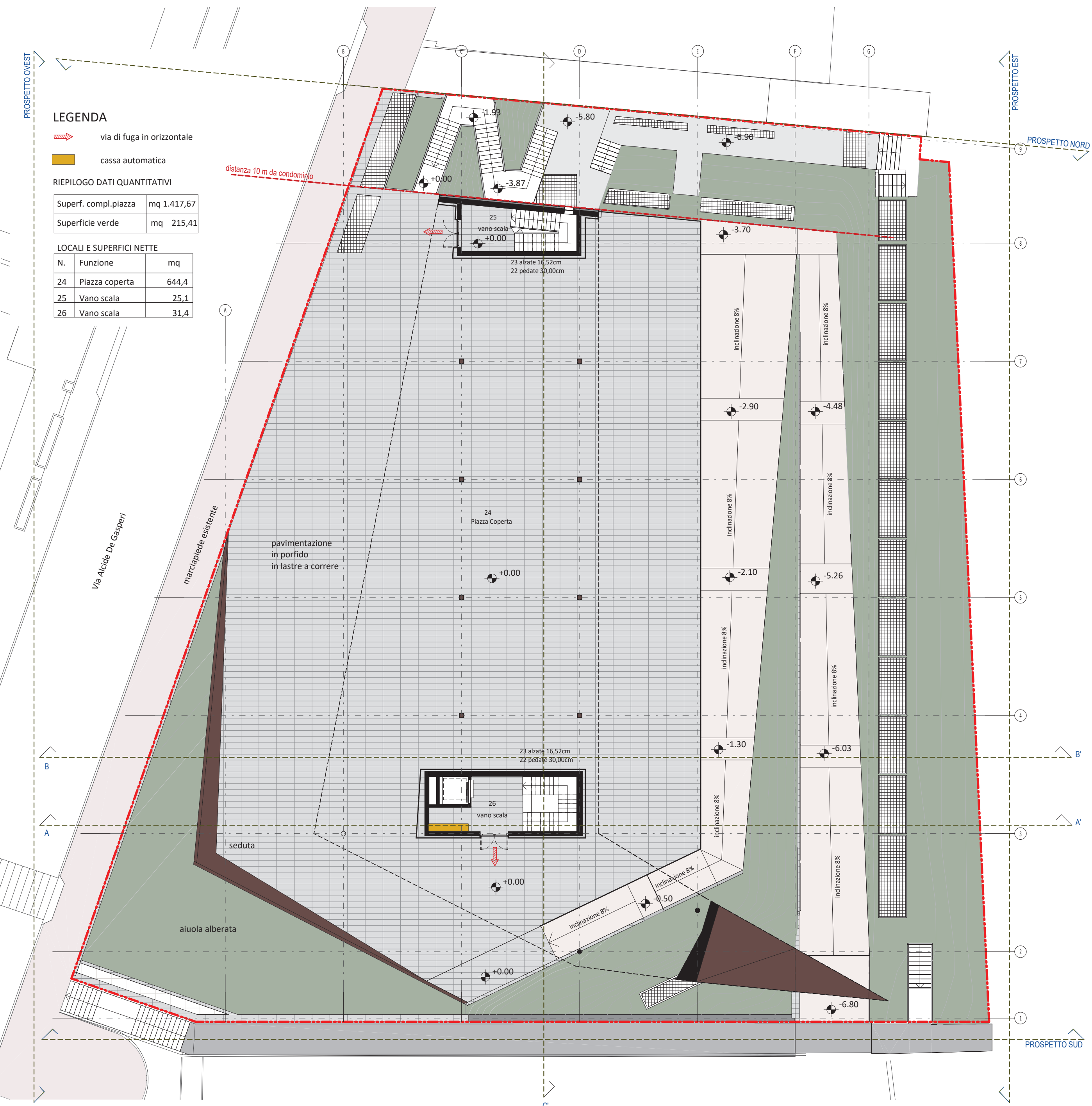
Pianta livello 0 scala 1:200
